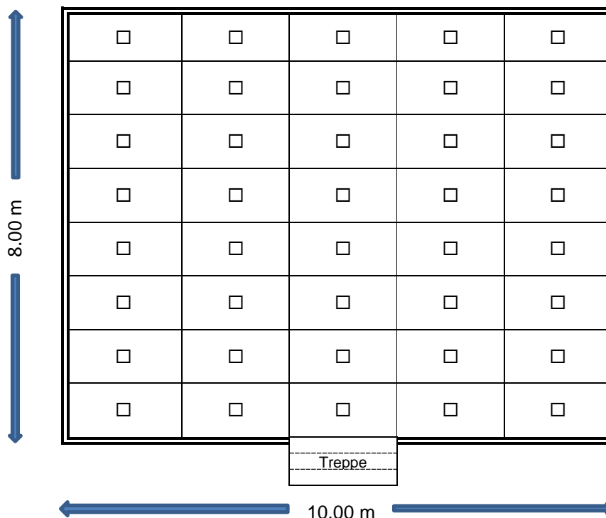
Skizze Bühnenelemente / 40 Elemente à 1 m x 2 m
